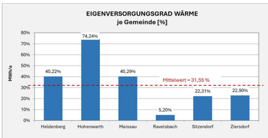
Abbildung 28 Eigenversorgungsgrad Wärme
