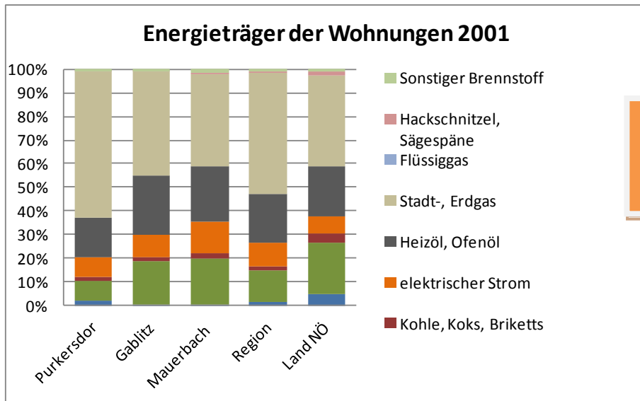
Abbildung 20: Energieträgereinsatz laut Gebäude und Wohnungszählung 2001
