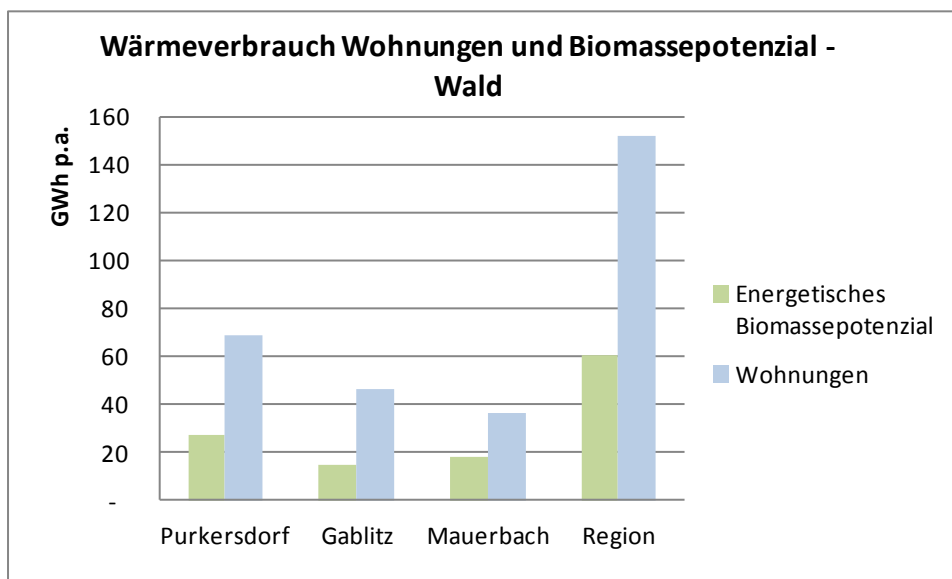
Abbildung 28: Wärmeverbrauch und Biomassepotenzial
