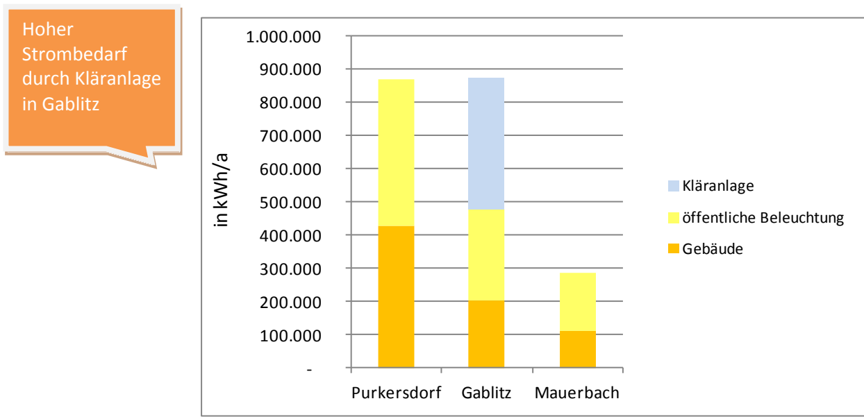
Abbildung 22: Strombedarf der Kommunen nach Einsatzzwecken
