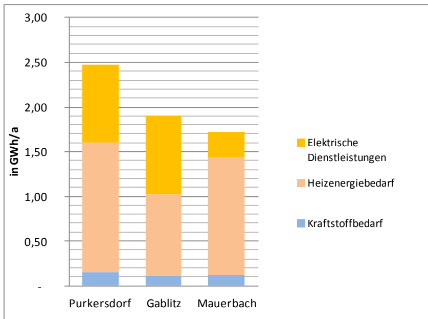
Abbildung 21: Energiebedarf der Kommunen
