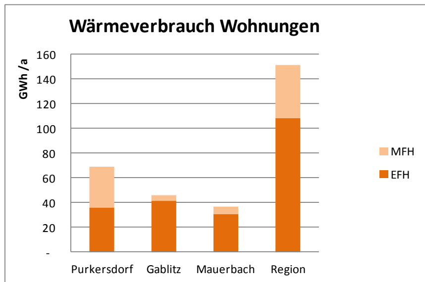
Abbildung 19: Wärmeverbrauch nach Gebäudetypen
