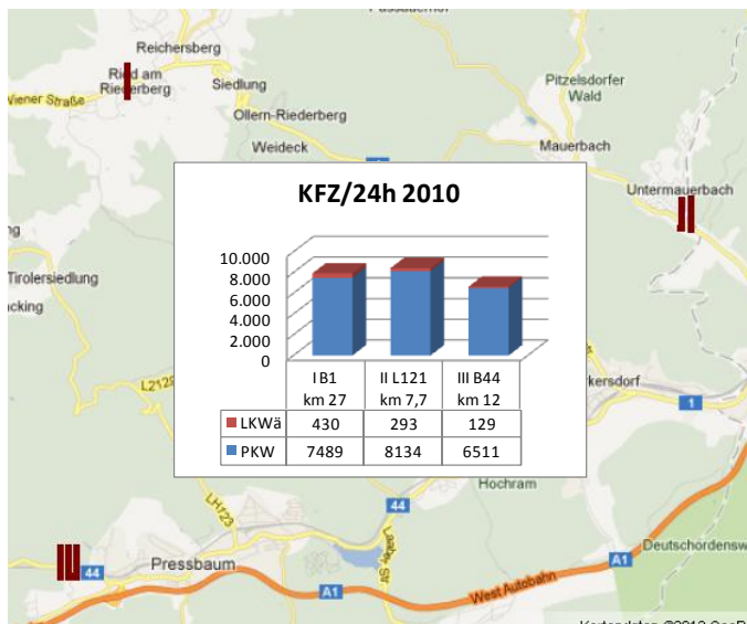
Abbildung 24: Standorte Verkehrszählungen und Ergebnisse 2010 (Land NÖ, 2012)
