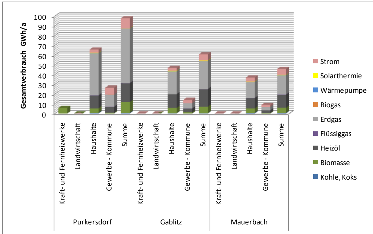
Abbildung 14: Energieträgereinsatz Wärmebereitstellung nach Sektoren (Energiekataster NÖ 2008)
