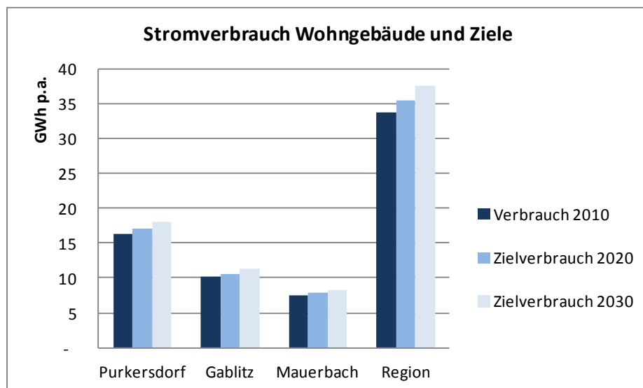
Abbildung 23: Stromverbrauch heute, Zielwerte 2020 und 2030
