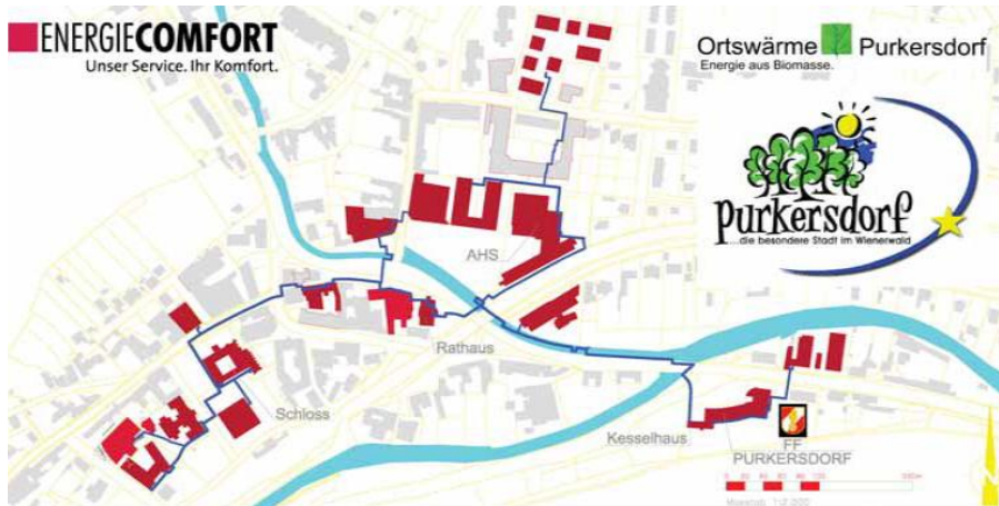
Abbildung 15: Biomassewärmernetz in Purkersdorf
