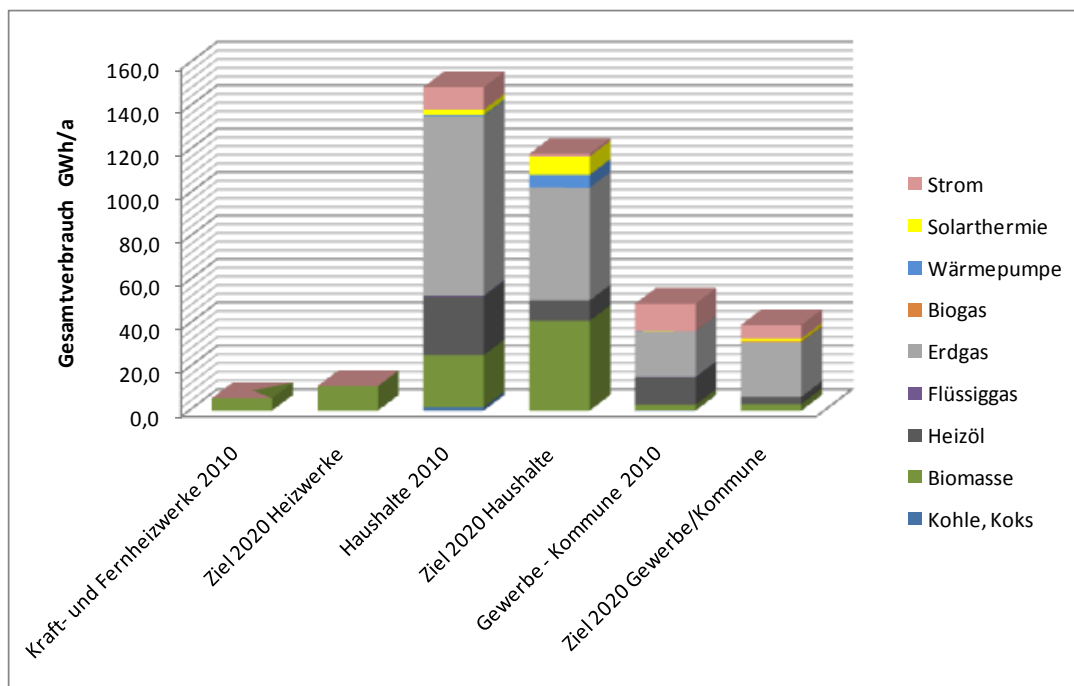
Abbildung 29: Gegenüberstellung Energieverbrauch (Wärme) 2010 mit Einsparzielen 2020
